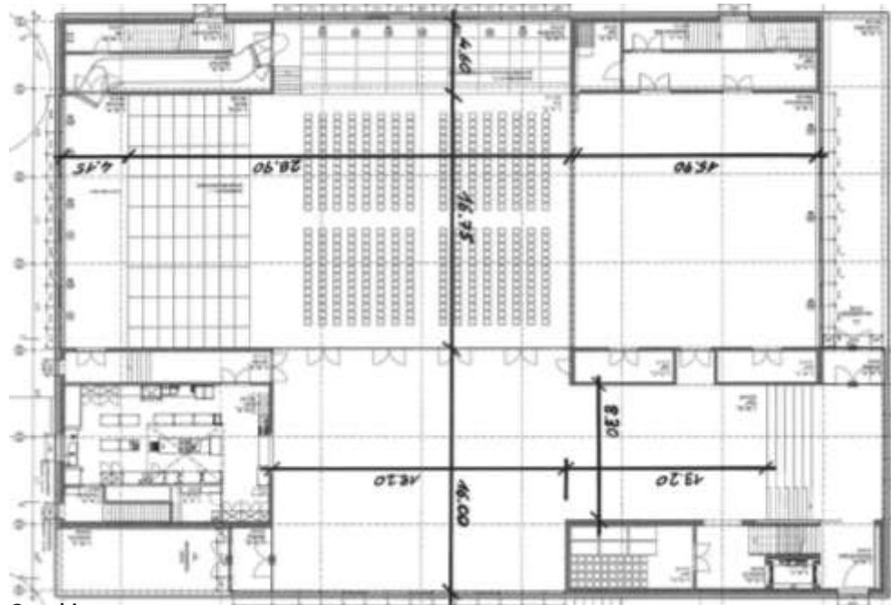
Grundriss
