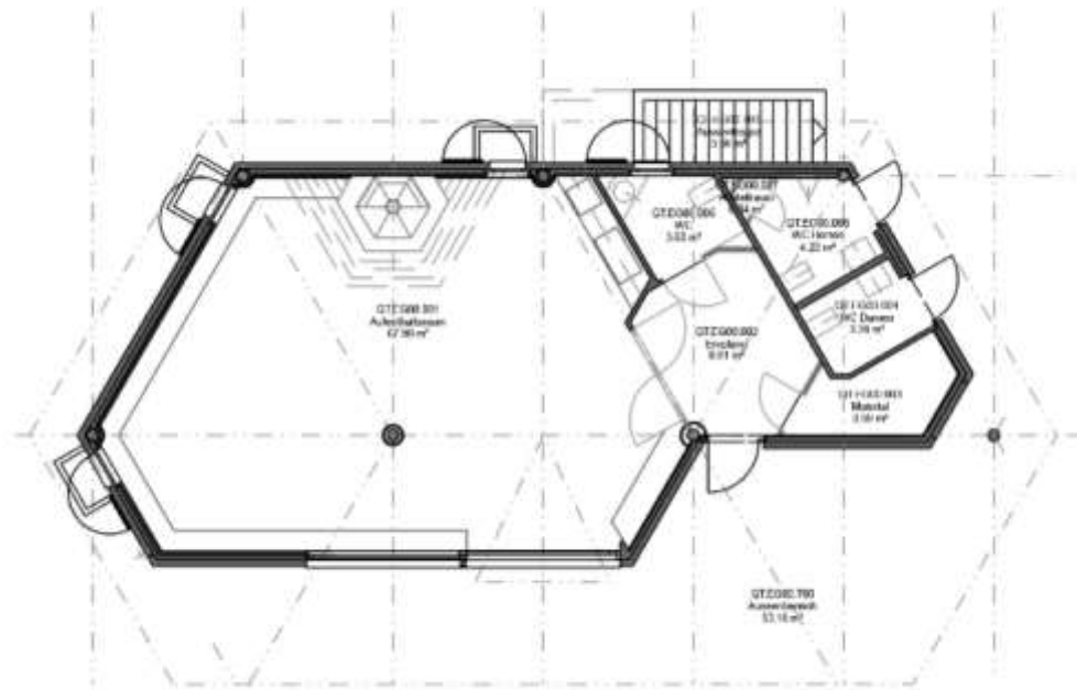
Grundriss Erdgeschoss
