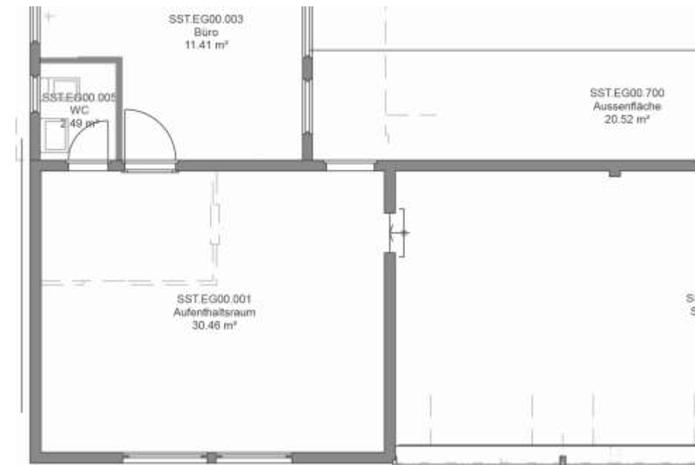
Grundriss Erdgeschoss
