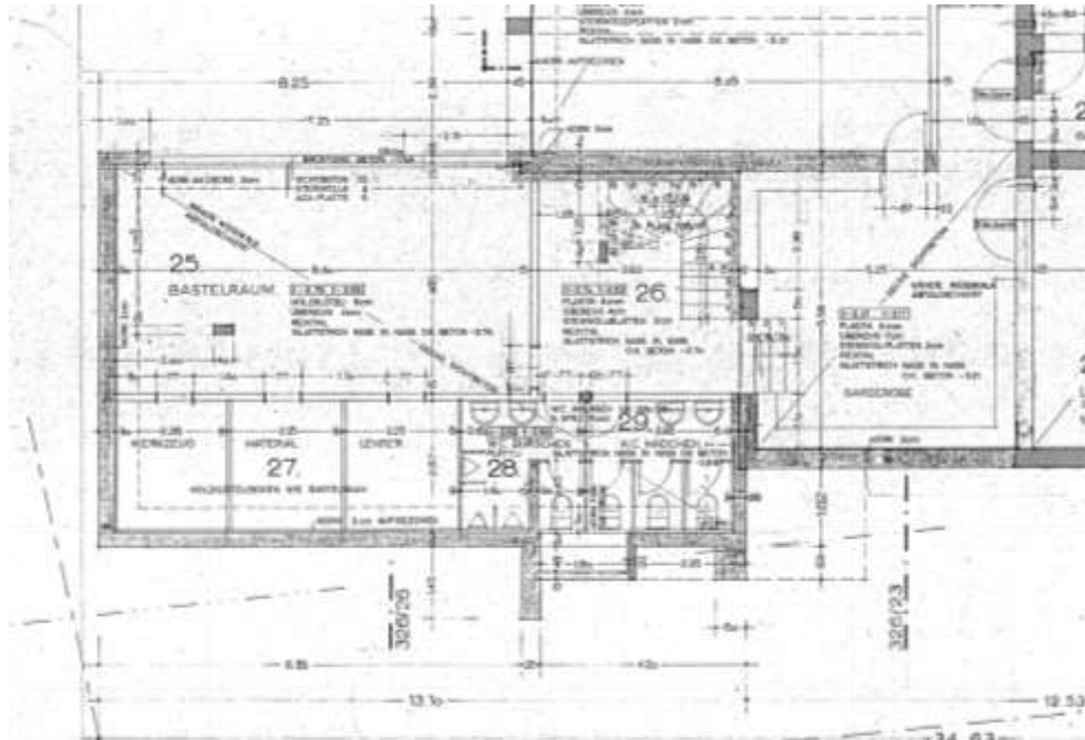
Grundriss Keller
