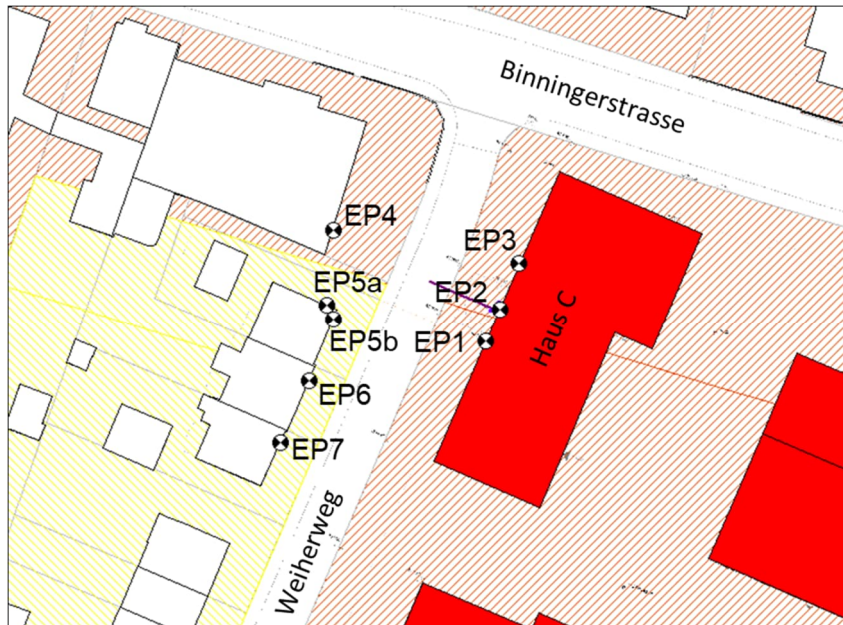
Abbildung 2: Lage der Immissionsorte (Industrie- und Gewerbelärm)
