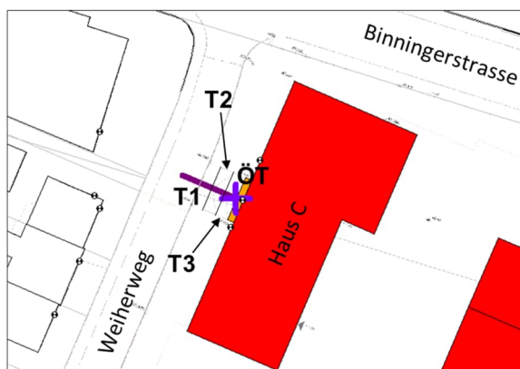
Abbildung 4: Lage der Lärmquellen
