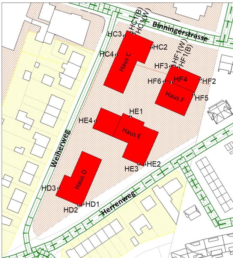
Abbildung 6: Lage der Immissionsorte (Strassenverkehrslärm)
